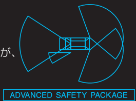
スバルリヤビークルディテクション (後側方警戒支援システム) 車体後部に内蔵されたセンサーにより、車の後側方から接近する車両を検知。ドミラーのインジケーターの点灯や点滅、ドライバーに注意を促します。また、後退支援時には警報音でも注意を促します。
