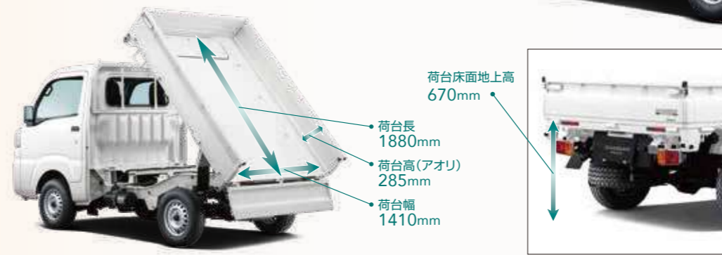
PHOTO:三方開ダンプ(4WD・AT車) ホワイトⅢ
