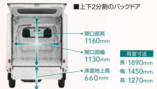
PHOTO:パネルバン ハイルーフ(4WD・AT車) ホワイトⅢ
