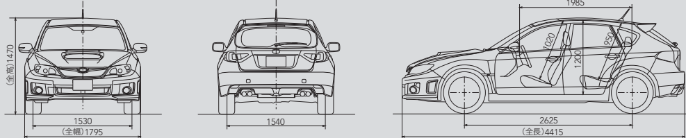
■ 3面図(WRX STI 5door) 単位:mm
